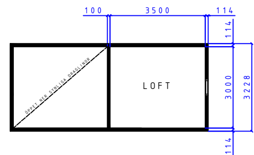
LOFTPLAN
