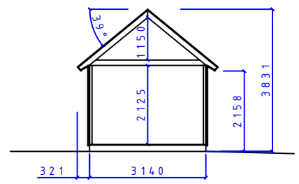
SEKTION A-A
