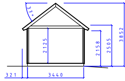
SEKTION A-A
