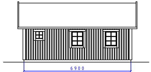
FASAD MOT
