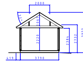
SEKTION A-A
