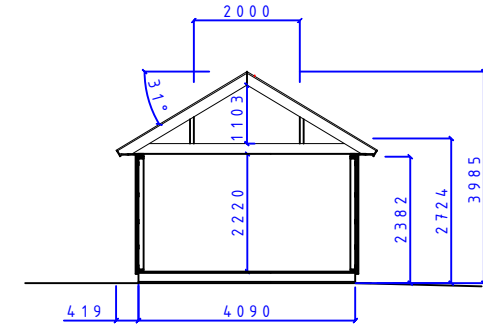
SEKTION A-A
