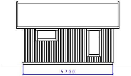
FASAD MOT
