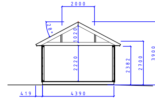
SEKTION A-A
