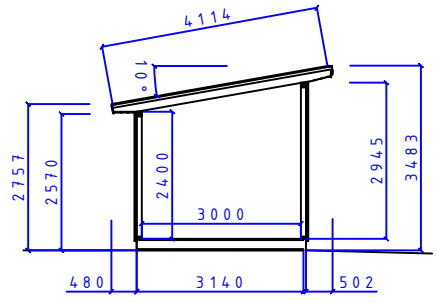
SEKTION A-A
