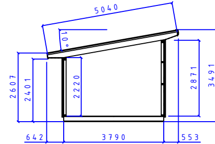
SEKTION A-A
