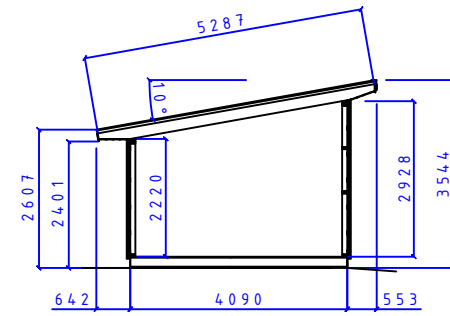
SEKTION A - A
