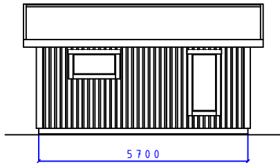
FASAD MOT
