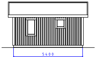
FASAD MOT
